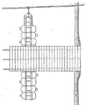
Fig. 288. — Passerelle de radeaux de sacs.
